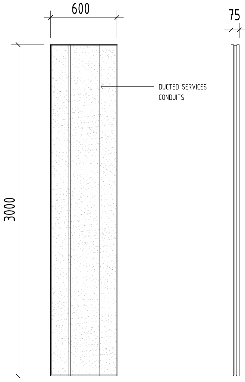
ELEVATION
